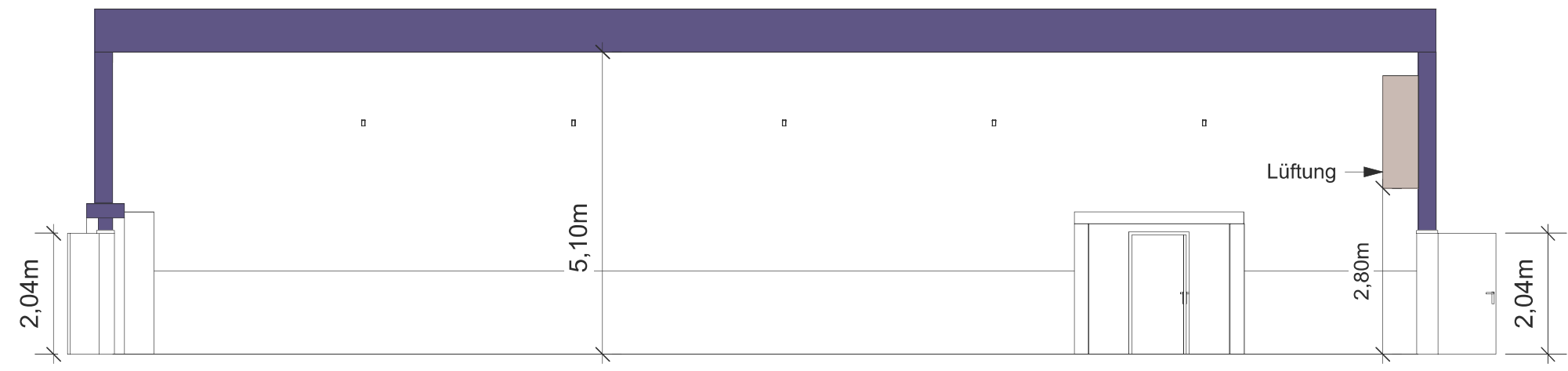
1 01 Längsschnitt Maßstab: 1:100
