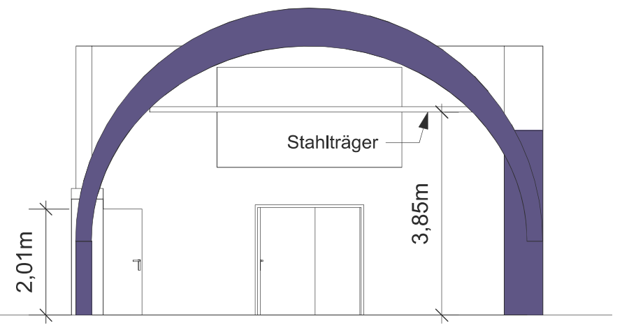
2 01 Querschnitt Maßstab: 1:100
