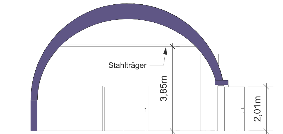
2 Querschnitt 01 Maßstab: 1:100
