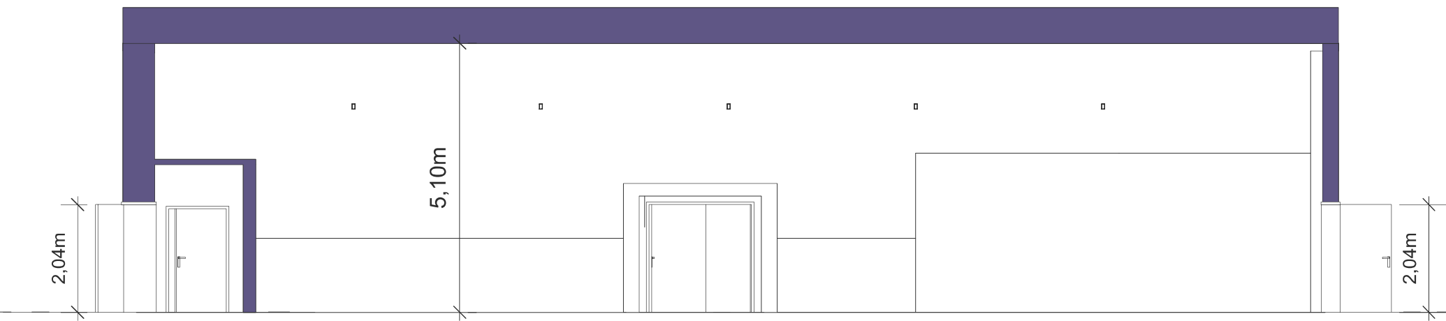
1 Längsschnitt 01 Maßstab: 1:100
