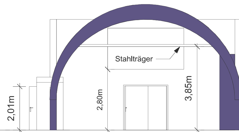
2 01 Querschnitt Maßstab: 1:100
