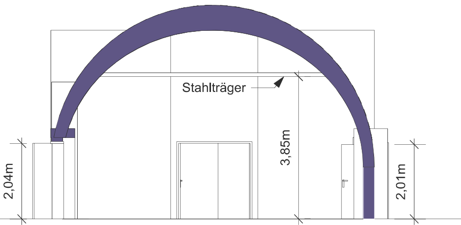
2 Querschnitt 01 Maßstab: 1:100
