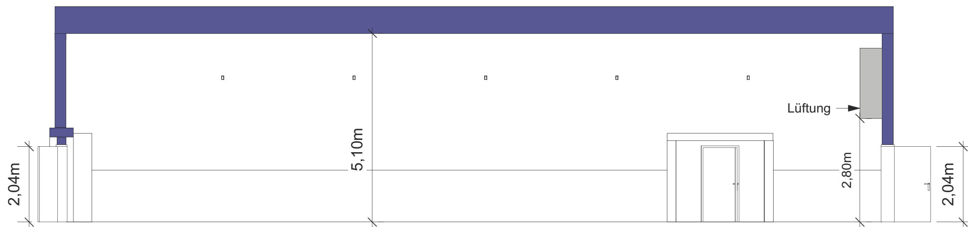
1 Längsschnitt 01 Maßstab: 1:100
