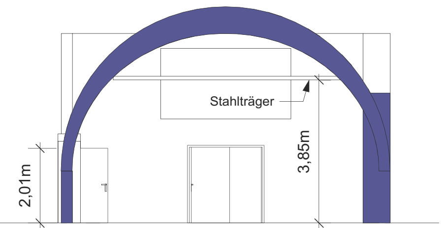
2 Querschnitt 01 Maßstab: 1:100
