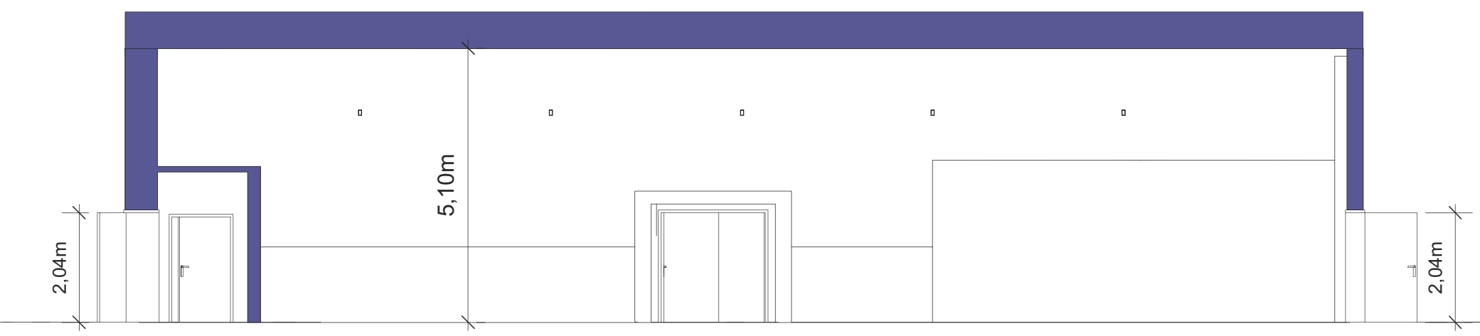
1 Längsschnitt 01 Maßstab: 1:100
