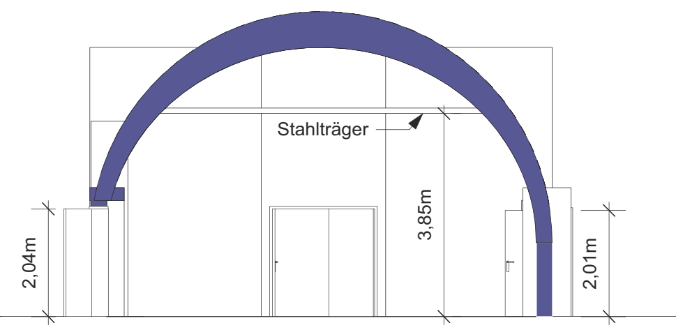
2 Querschnitt 01 Maßstab: 1:100
